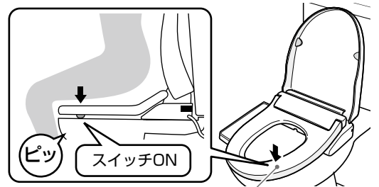
着座スイッチ (便座裏面)
